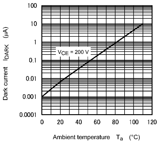
Fig. 11.9 I_{DARK} - T_a
