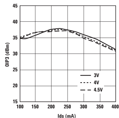
Figure 28. OIP3 vs I_{ds} and V_{ds} at 3.9 GHz.
