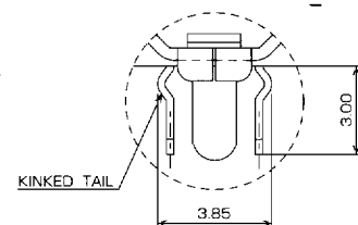
P/N : HSB-ARB62-T 3 15A
