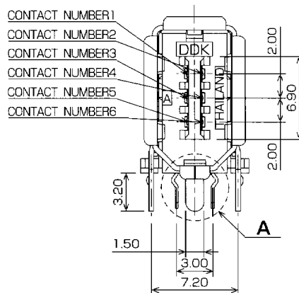
P/N : HSB-ARB62-T 3 15A
