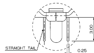
Detail A P/N : HSB-ARB62-T 2 15A
