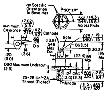
JEDEC Outline TO-48
