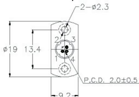
FC Receptacle
