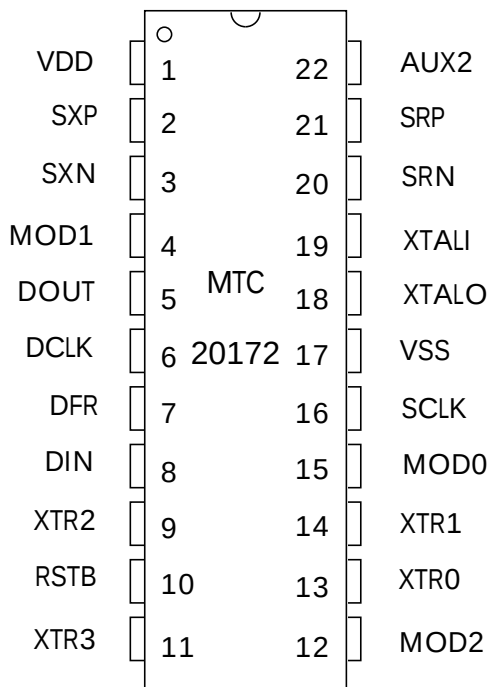
Fig. 2.9 : Pin Descriptions
