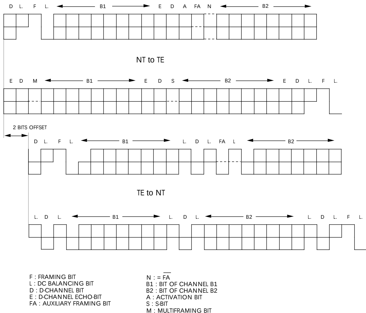
Fig. 2.5 : So-Frame Format
