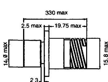
MC400E-* -09-02 ** Receptacle
