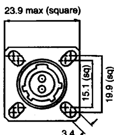
MC400E-* -09-02 ** Receptacle
