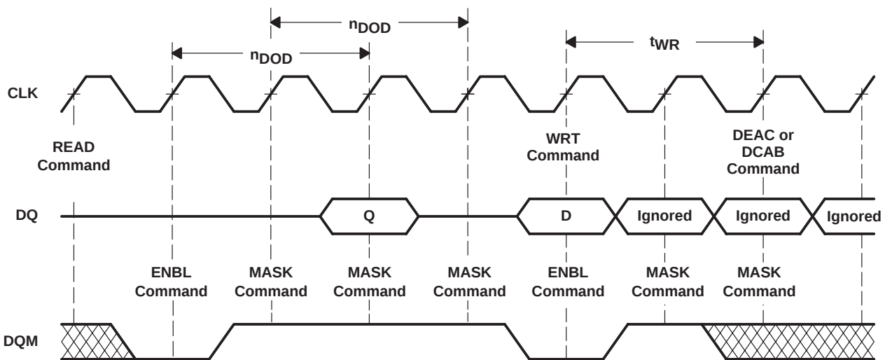
Figure 16. DQ Masking
