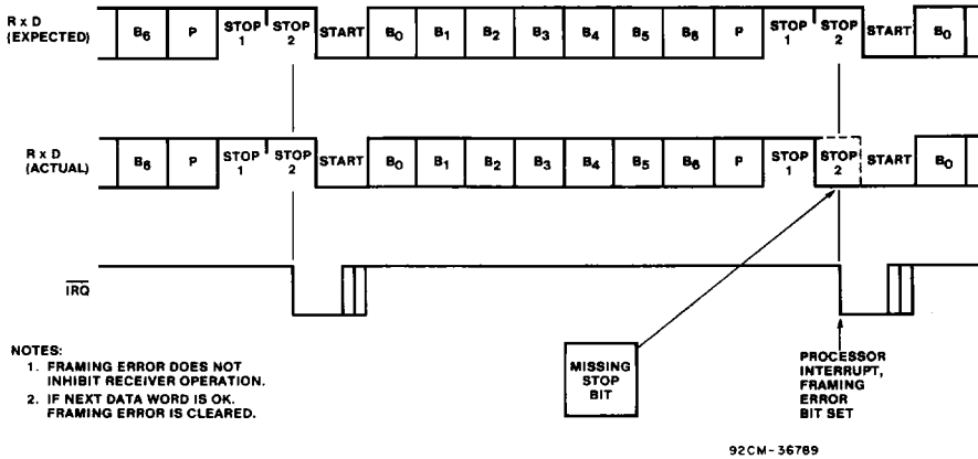
Fig. 16 - Framing error.
