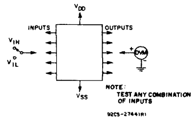
Fig. 16 - Input voltage.
