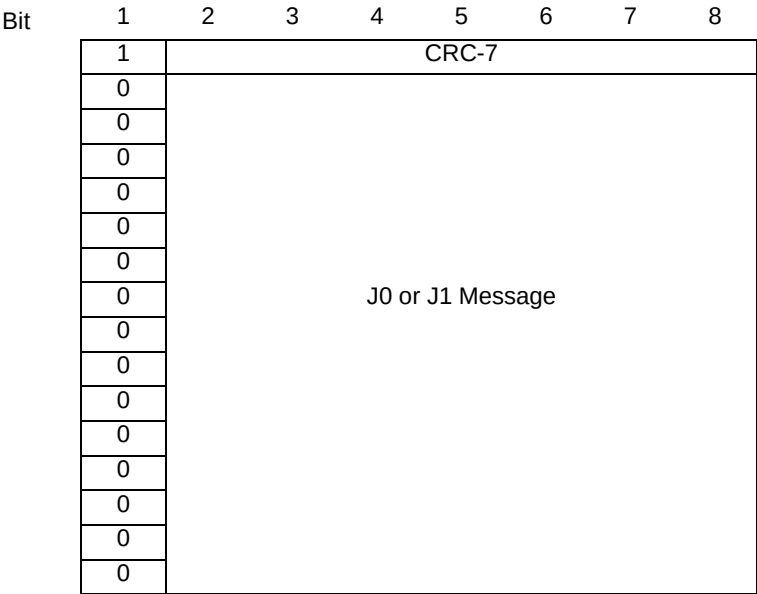
J0/J1 Message Format
