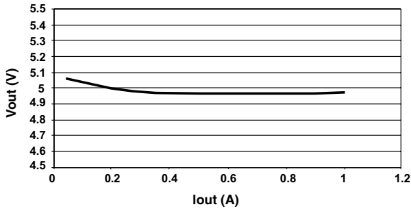
Vout Vs. Iout* Vin = 3.5V; Vout = 5.0V
