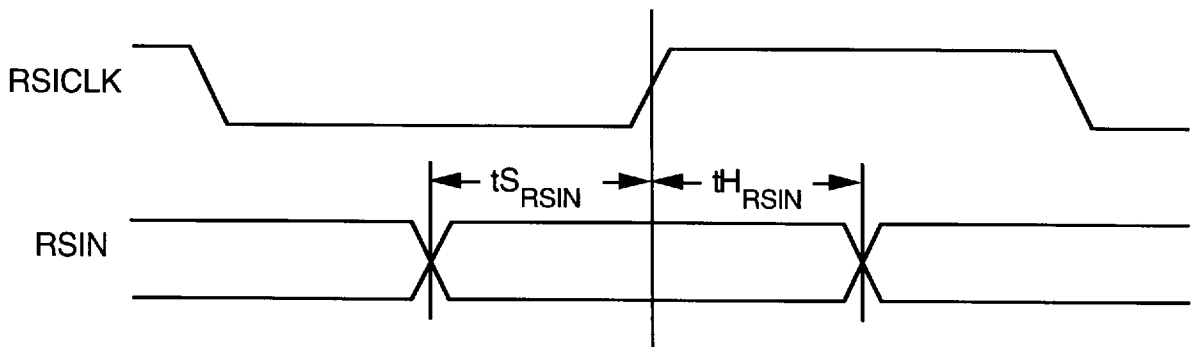
Fig. 30 STS-1 Input
