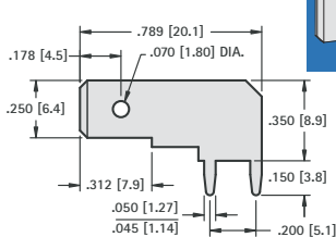
.250 (6.4) TAB
