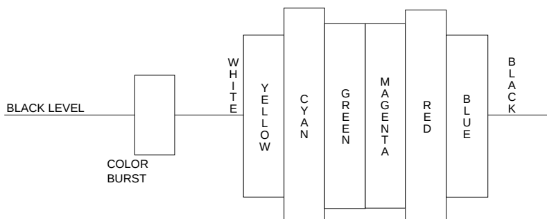
Fig. 9 COUT output
