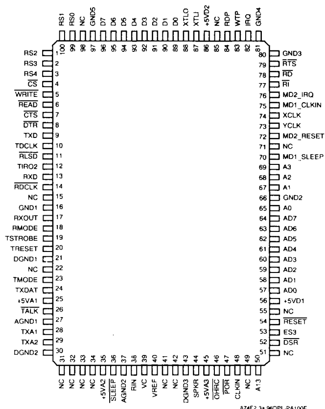
a. 100-Pin PQFP
