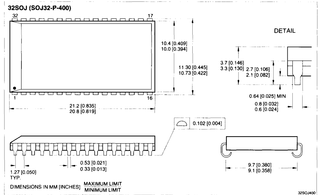
32-pin, 400-mil SOJ
