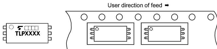
Fig. 17.3.1.1 Device Orientation
